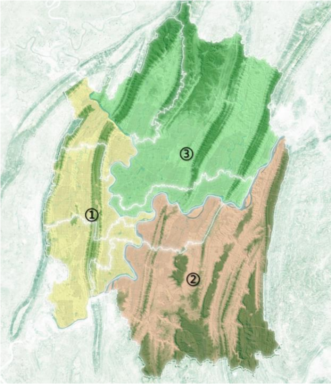
图 1.7-1 中心城区暴雨强度公式分区
