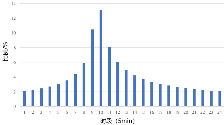
图 3.1-4 中心城区 2 小时设计暴雨雨型
