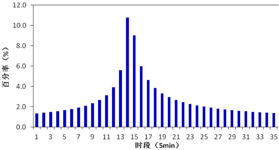
图 4.3-2 3 小时设计暴雨过程
