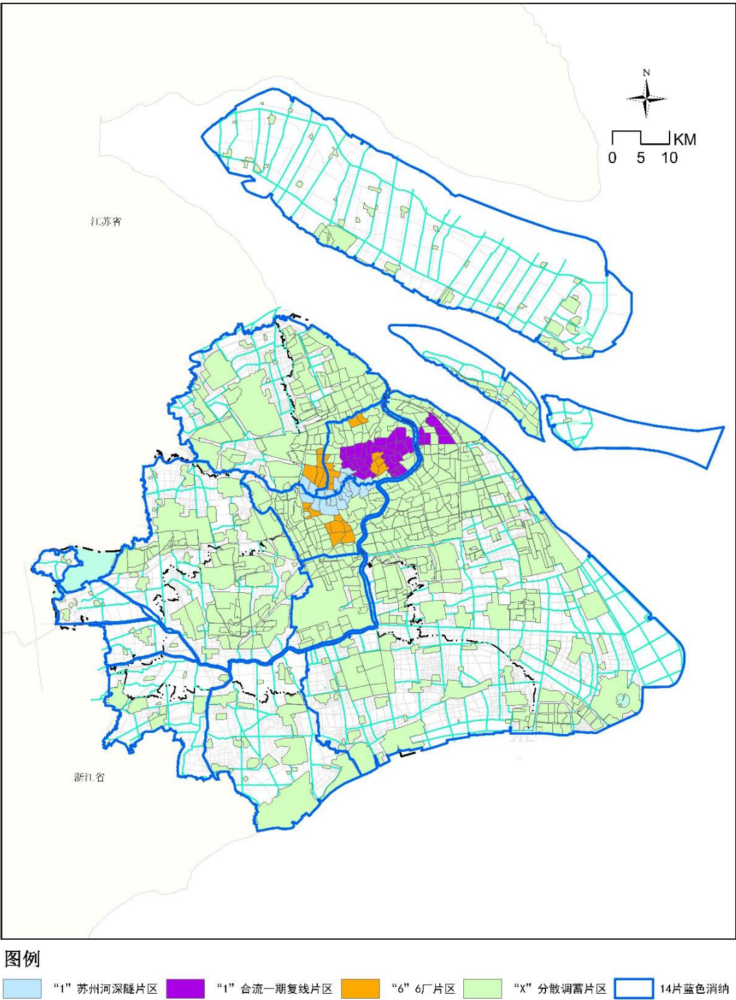
图 4.1-7 上海市城镇雨水排水规划布局图
