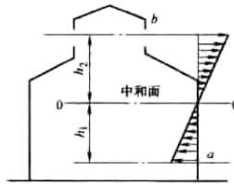
图 2 余压沿建筑高度的变化
