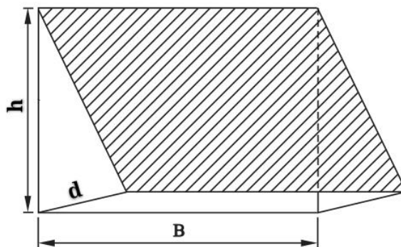
图 3 悬开窗通风开口有效面积计算示意图
