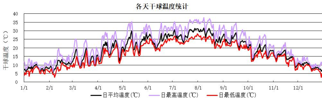
图 1 重庆地区全年日干球温度
