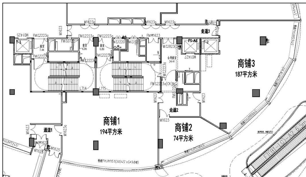
图 1 建筑平面图
